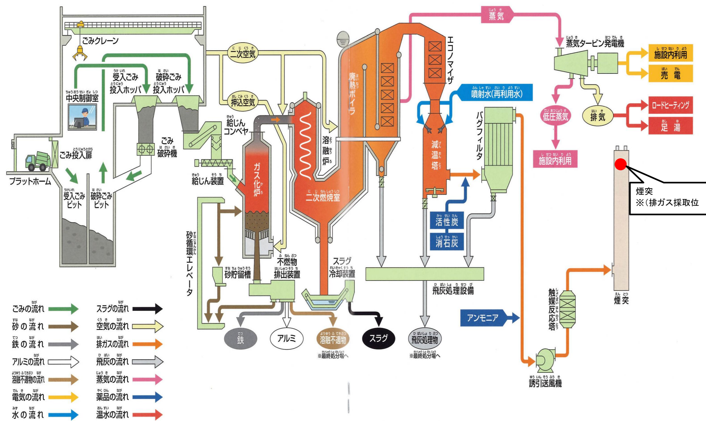
エネルギー回収施設(川口)における排ガスの採取位置図
